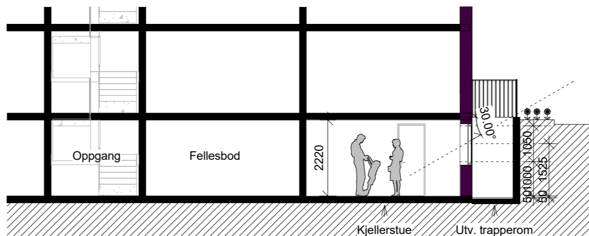
Snitt A-A 1 : 100
