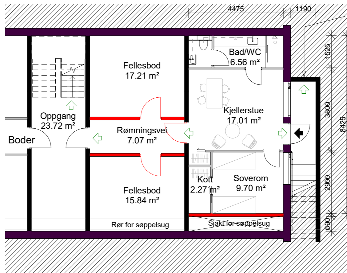
Plan Hybel 1 : 100
